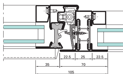
Herraje para ventana oculto
